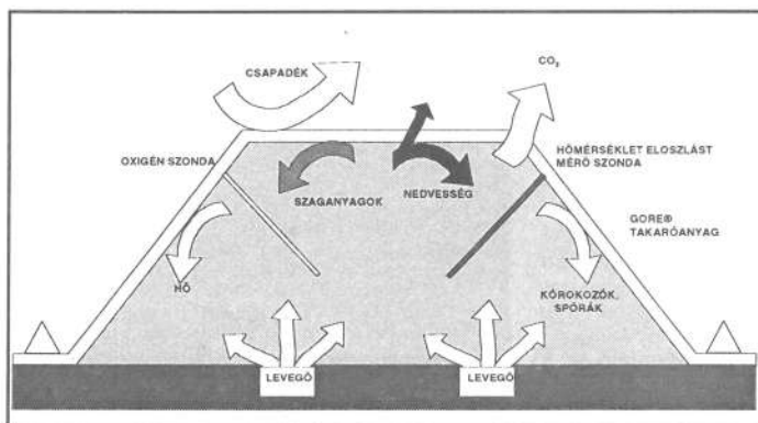
A komposztáló prizma működési elve
